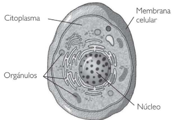
Figura 20. La célula como un microchip. Como un cristal semiconductor.
