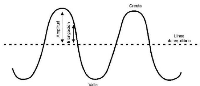
Figura. Características de una onda.
